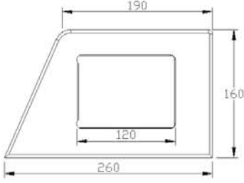
Ford Otosan Ayak Basamağı Foot Step
