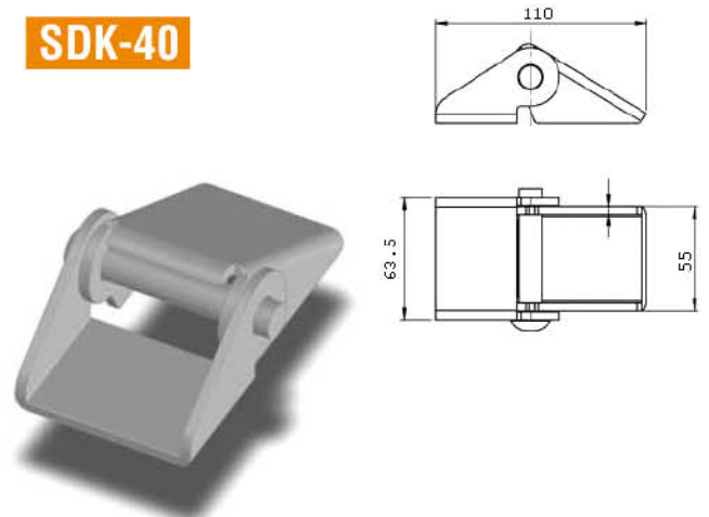
Orta Boy Damper Menteşesi (5 mm) Middle Size Dumper Hinge (5 mm)
