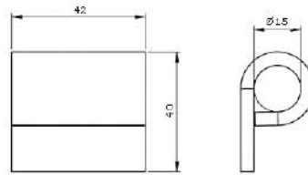
Kısa Bacaklı Boru
