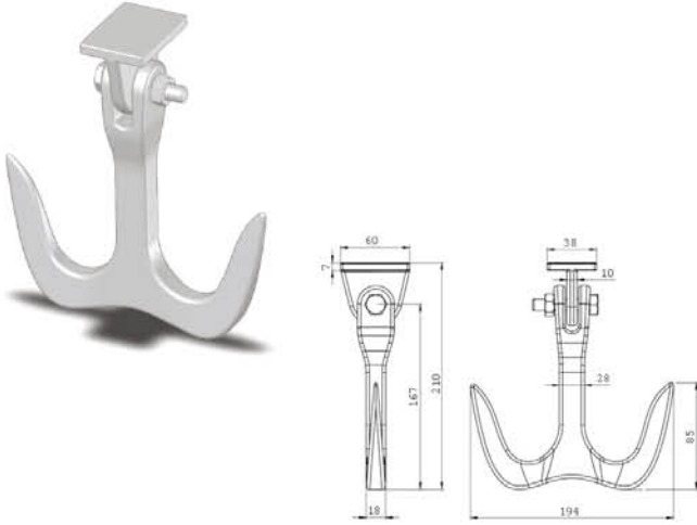
Çiftli Et Kancası Kod SDK907 Meat Hook Code SDK907
