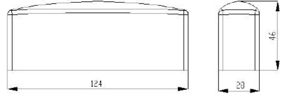
Plastik Tahtalık Başlığı Kod SDK340 Plastic Cap Code SDK340
