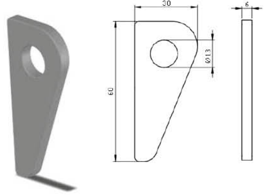
Orta Boy D Tipi Menteşe Middle Size D Type Hinge
