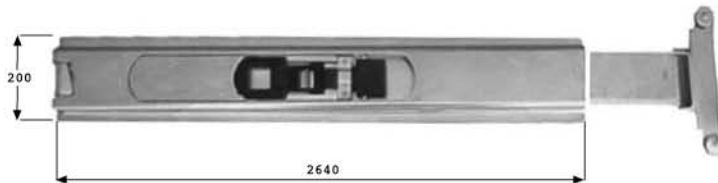
Kayar Baba Plastikli Kod SDK781 Sliding Pillar Code SDK781
