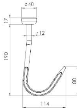
Paslanmaz Tekli Et Kancası SDK911 Stainless Steel Meat Hook SDK911
