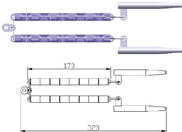
Yuvarlak Çiftli Hortumlu Kama Round - Double Chain Pin
