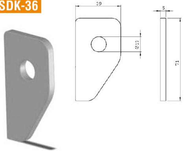
Aydın Tipi Büyük Menteşe Big Hinge
