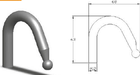
12 mm Bagaj Kancası 12 mm Hook
