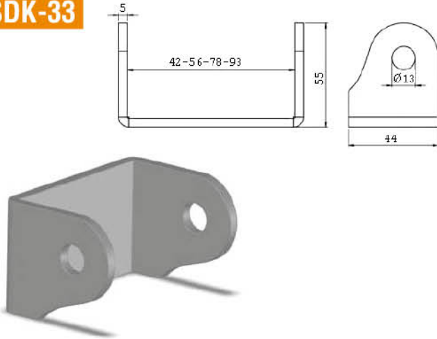
U Menteşe U Hinge
