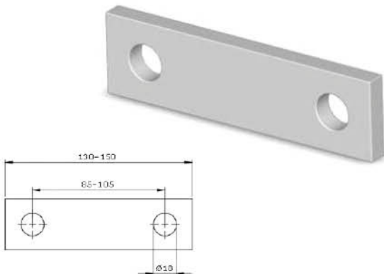
Bağlantı Kepli Cap of Connection Fixing
