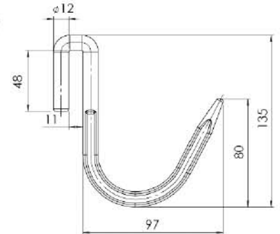
Paslanmaz Et Kancası Yan SDK910 Stainless Steel Meat Hook SDK910
