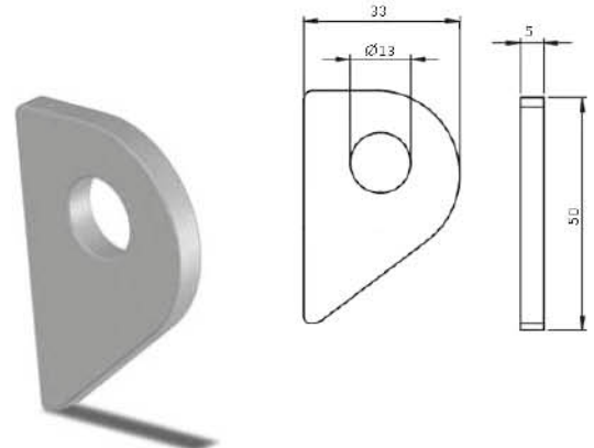
Konya Tipi Küçük D Menteşe Small D Hinge
