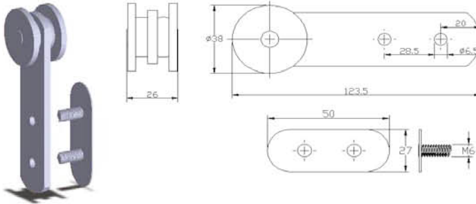
Perde Makarası Sliding Curtain Runner
