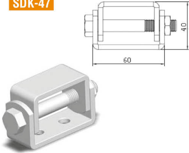
Ford Otosan Mentşe | Ford Otosan Hinge
