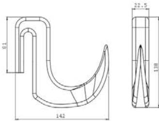
Yan Et Kancası Kod SDK909 Meat Hook Code SDK909
