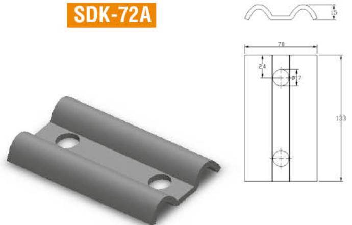
Bağlantı Kepli Cap of Connection Fixing
