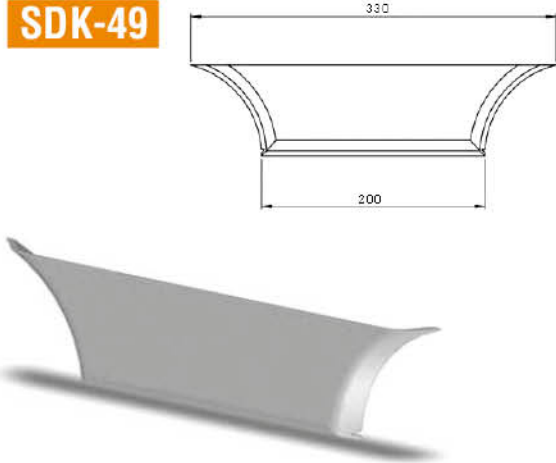
Köşeli Etek Sacı | Metal Sheet Belt (Cornered)
