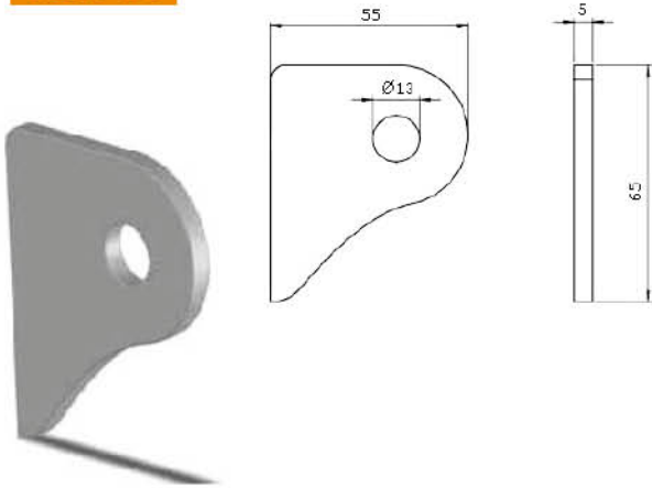
Konya Tipi Büyük D Menteşe Big D Hinge
