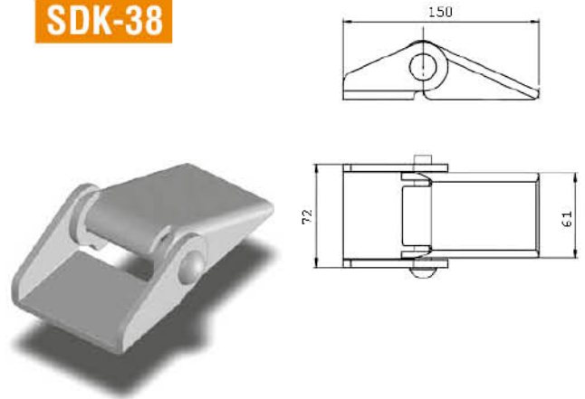
Büyük Damper Menteşesi Big Dumper Hinge
