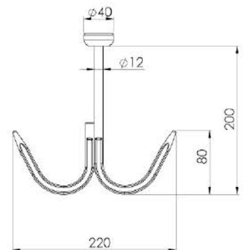
Paslanmaz Çiftli Et Kancası SDK912 Stainless Steel Meat Hook SDK912
