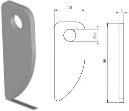
Büyük D Tipi Menteşe Big D Type Hinge
